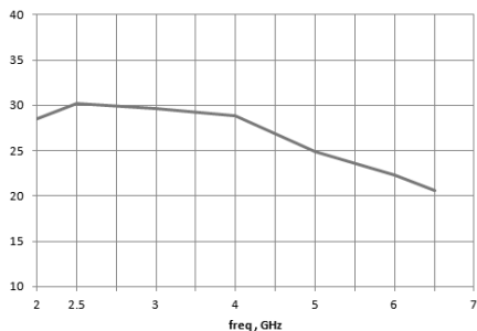
小信号增益
